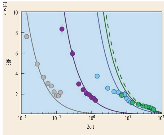
Abb. 2 Der sog. Ergodizitäts-Bruchparameter (EBP) gibt an, wie weit sich die Ausbreitung mit zunehmender dimensionsloser Zeit vom ergodischen Gauß-Zustand unterscheidet. Er fällt langsam ab, invers proportional zur Flugzeit 1/t . Die Geschwindigkeit seiner Konvergenz gegen Null hängt jedoch von den gewählten Parametern des Experiments ab.
