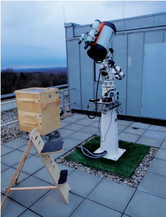
Abb. 4 Mit wenigen Handgriffen lässt sich das Teleskop aufsetzen, Strom und EDV-Anschlüsse sind schnell hergestellt. Links hinten ist der Zubehörowagen zu sehen, der u. a. den Teleskopaufsatz enthält sowie weiteres Material.
