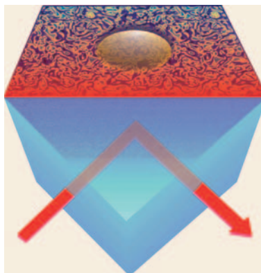
Abb. 1 Die kritische Casimir-Kraft, die durch Fluktuationen in einem Flüssigkeitsgemisch zwischen einer Kugel und einer Wand entsteht, beeinflusst die Bewegung der Kugel. Diese lässt sich durch die Totalreflexion eines Lasers an der Platte sehr genau bestimmen, da der Streubeitrag der Kugel exponentiell von ihrem Abstand abhängt.
