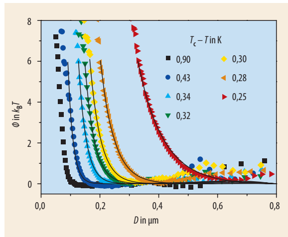
Abb. 2 Die kritische Casimir-Kraft bzw. das zugehörige Potential \Phi(D) werden umso größer, je stärker sich die Temperatur T dem kritischen Wert T_c annähert, an dem sich die Flüssigkeiten entmischen. Die durchgezogenen Linien zeigen die Ergebnisse der Theorie.
