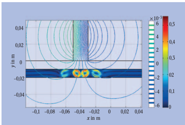
Abb. 2: Die Lösung des Problems zur Zeit t = 0,45 s. Der Surface-Plot zeigt das Geschwindigkeitsfeld (rechte Skala, in m/s), der Contour-Plot das Vektorpotential (linke Skala in Vs/m).
