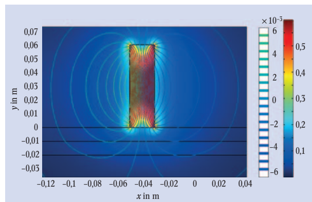
Abb. 1: Die mag. Flussdichte (Surface-Plot, rechte Skala in T) und das Vektorpotential (Contour-Plot, linke Skala in Vs/m).
